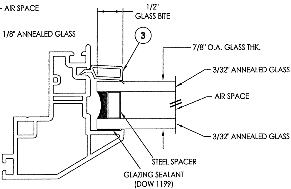
G2 GLAZING DETAIL
