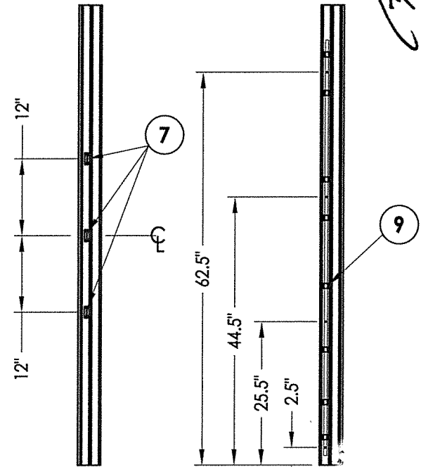
HINGE JAMB
